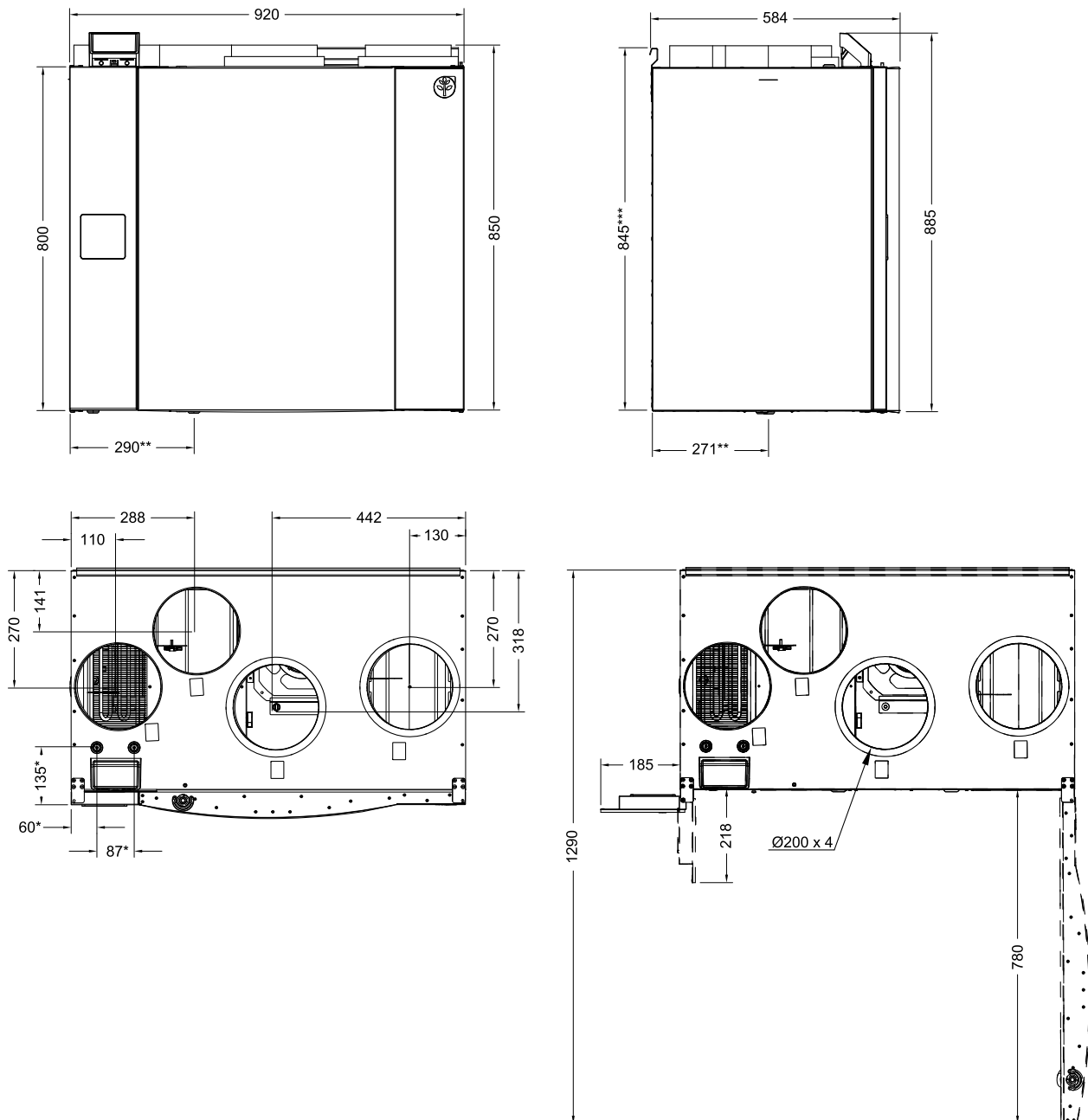
Pav. 2 Matmenys ir svoris, L modelis
